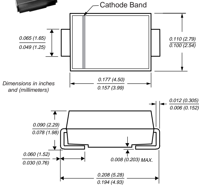
DO-214AC (SMA)
